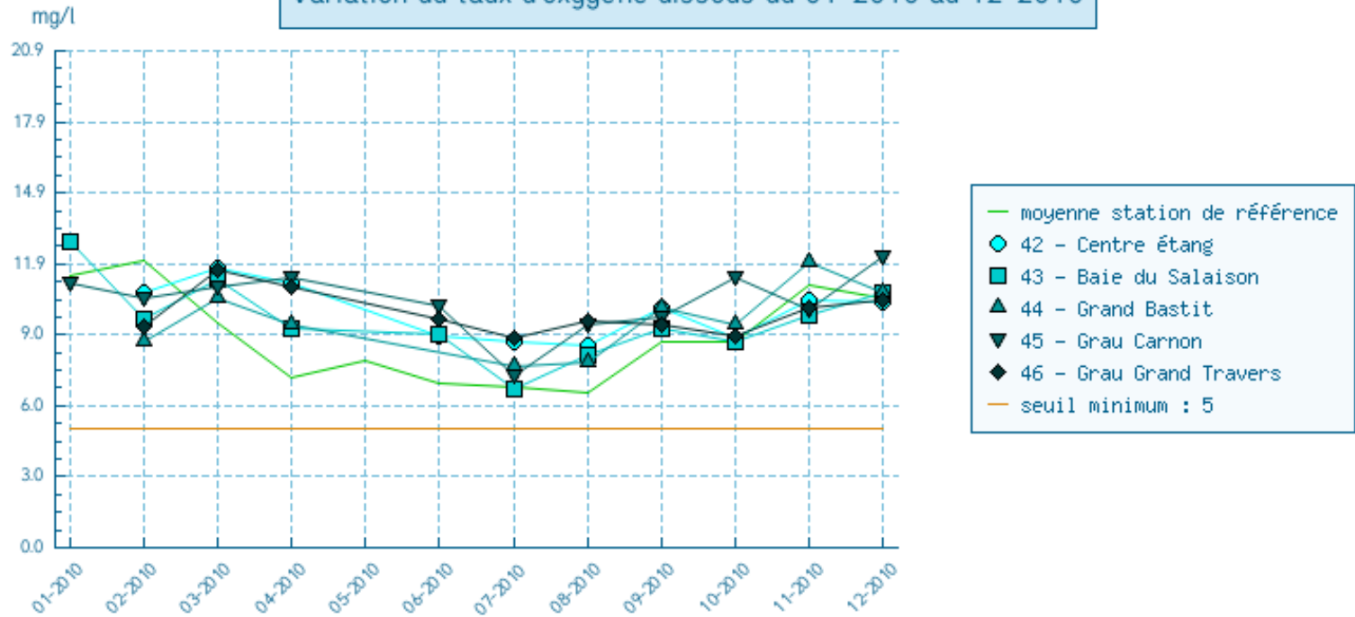
Variation du taux d'oxygène dissous du 01-2010 au 12-2010
