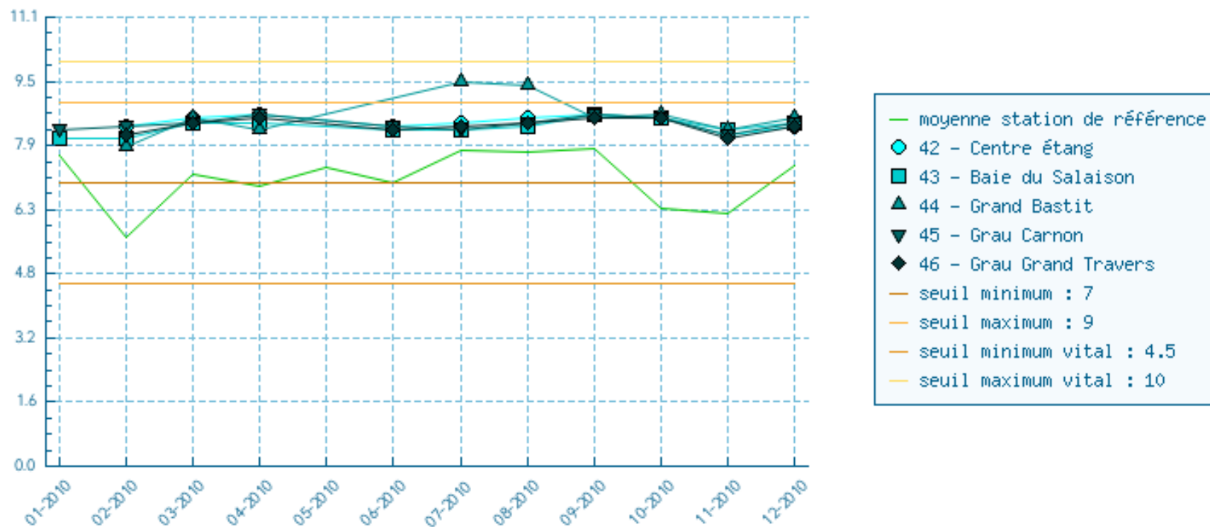
Variation pH du 01-2010 au 12-2010
