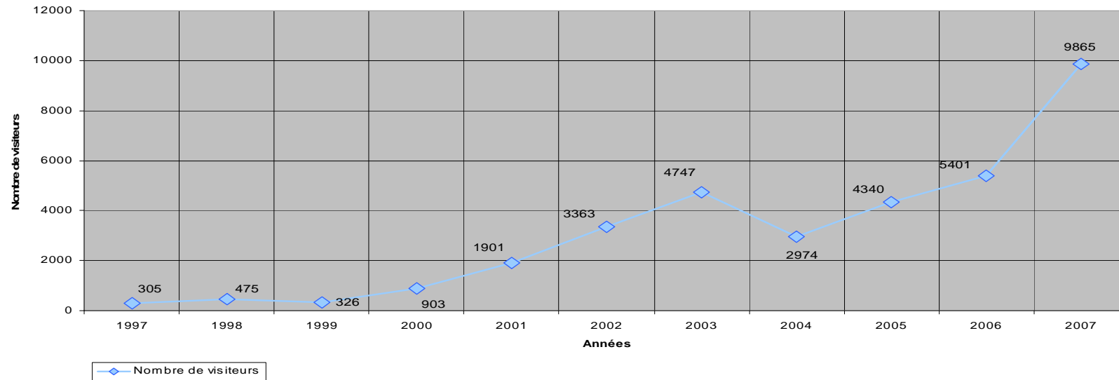
Evolution fréquentation 1997 → 2007
