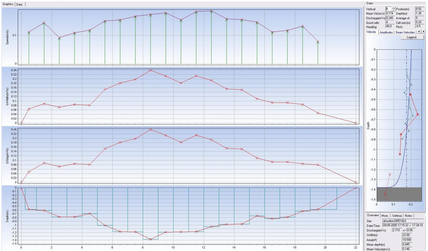
Figure 3: Principe de mesure du profileur à effet acoustique; division d'une section en plans verticaux; Exemple de résultat sur le terrain à l'Afoux du Lion (passe entre l'étang du Vaccarès et l'étang du Lion)
