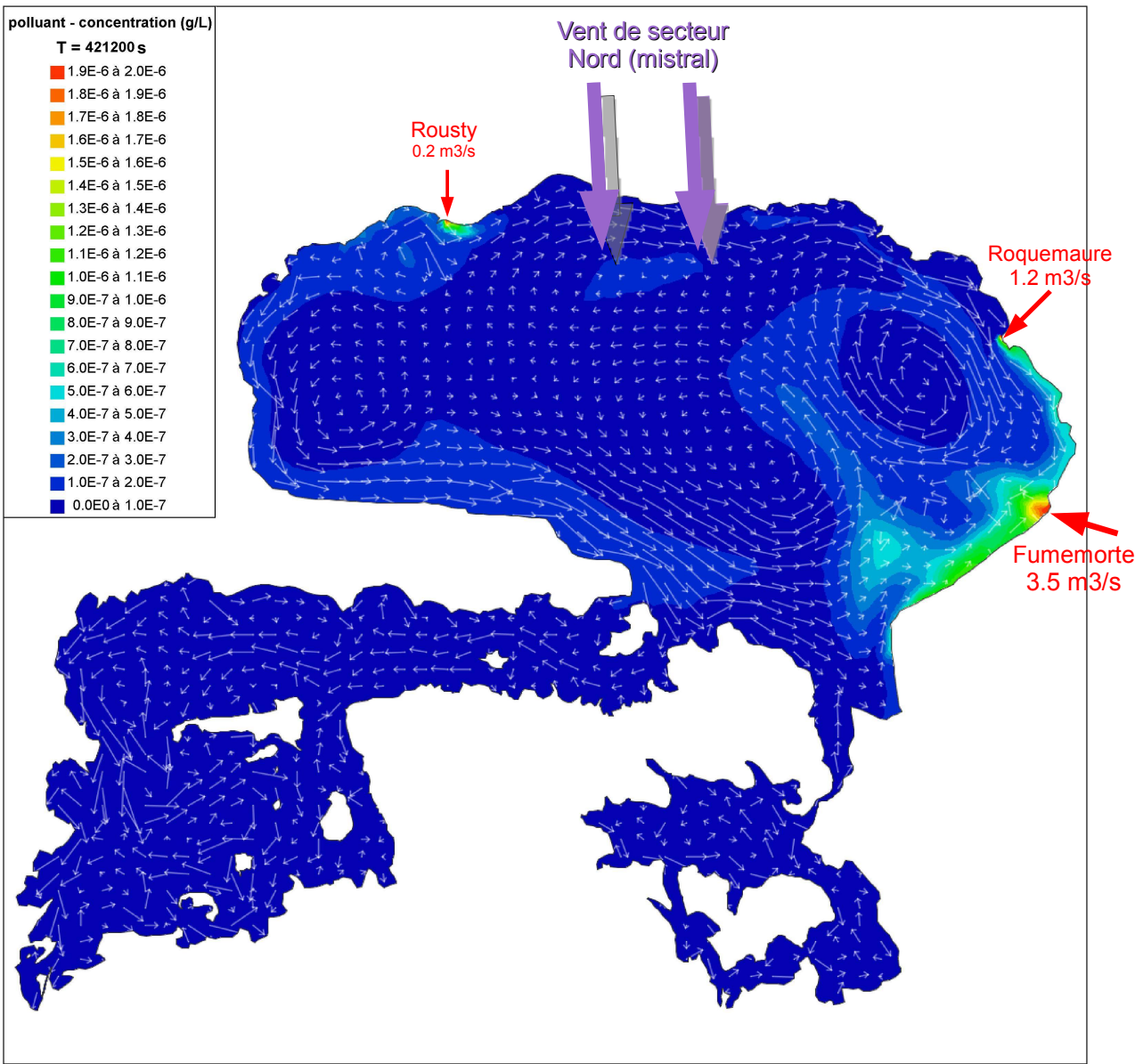
Figure 4: Fin de simulation hydrodynamique de la période allant du 19 au 24/06/2009; Vent réel; concentration hypothétique de polluant (pesticides) égale à 2µg/L dans chaque canaux de drainage; débit constant durant toute la simulation
