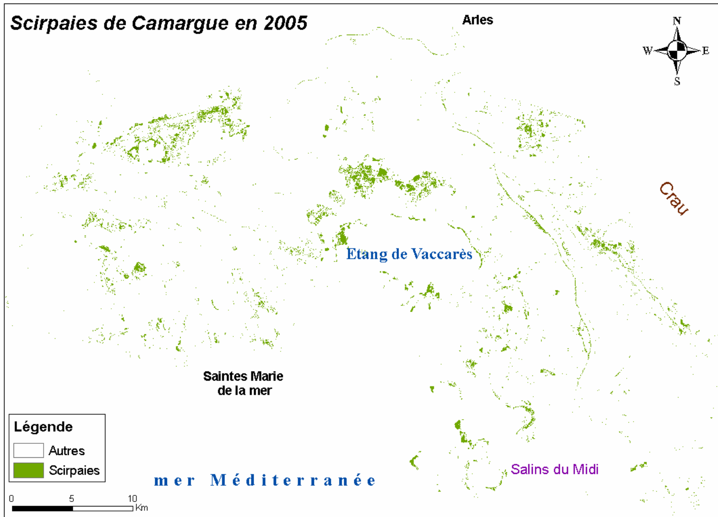
Figure 50 : Cartographie des scirpaies de Camargue en 2005 obtenue par application de la formule de classification de la présence de scirpaies aux images satellitales de l'année 2005
