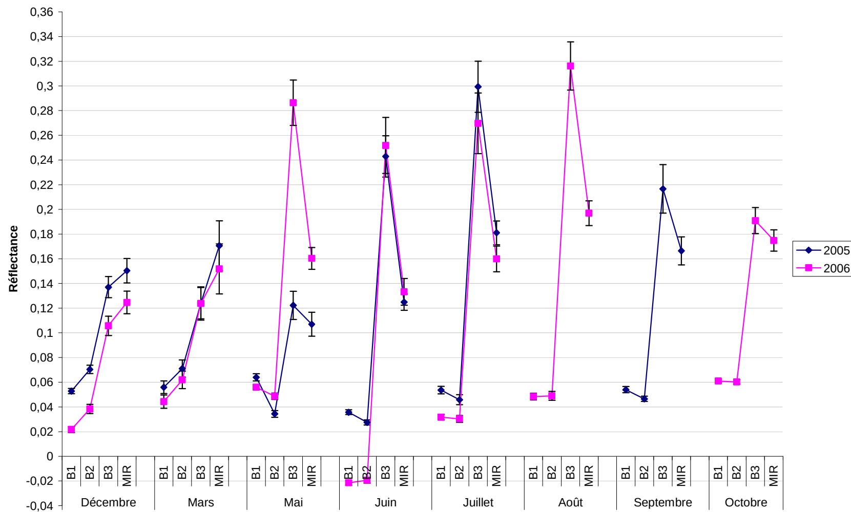
Figure 20 : Variation quasi-annuelle de la réflectance des phragmites en Camargue. Les barres d'erreur représentent les intervalles de confiance à 5% ( 1.96 \cdot SE )
