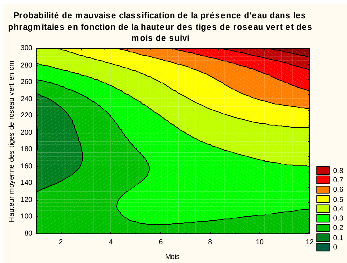
Figure 55 : Paramètres pouvant influencer la classification de la présence d'eau dans les phragmitaies
