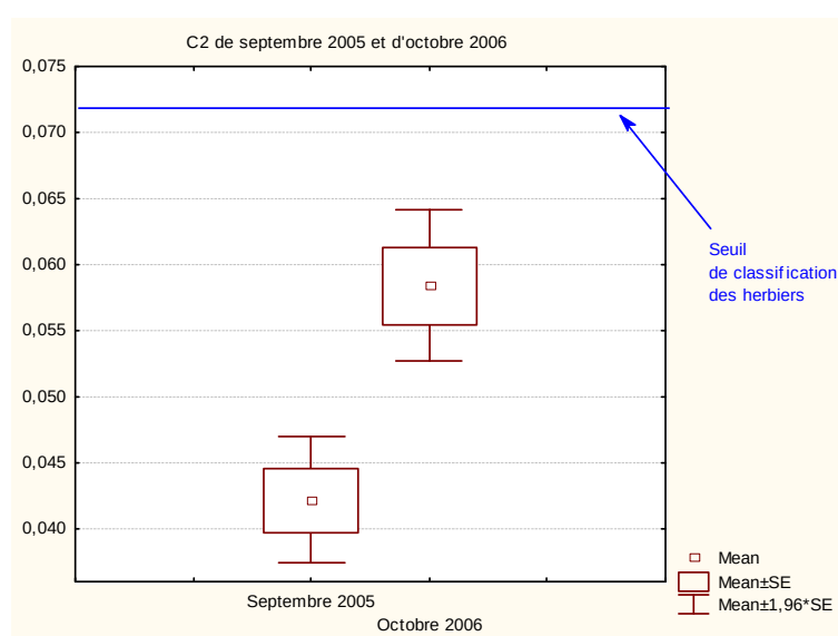
Figure 37 : Comparaison de la variable c29 calculée pour les années 2005 et 2006 à partir des données de radiométrie des échantillons d'herbiers aquatiques des marais permanents typiques de domaines privés ( t=-5.76 , p=0 )
