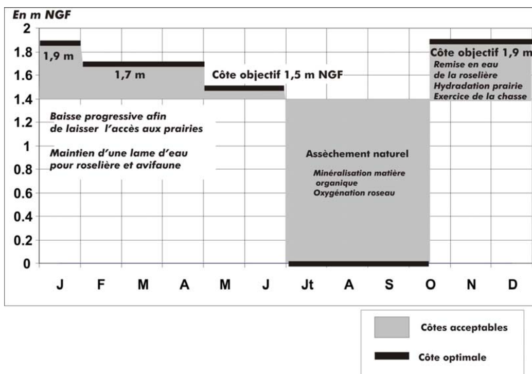
Schéma simplifié des objectifs de gestion des niveaux d'eau (ouvrage Canal de la Matte)
