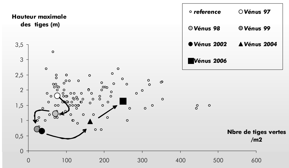
Fig. 2 : Evolution de la qualité de la roselière de l'étang de Vendres 1997-2007
