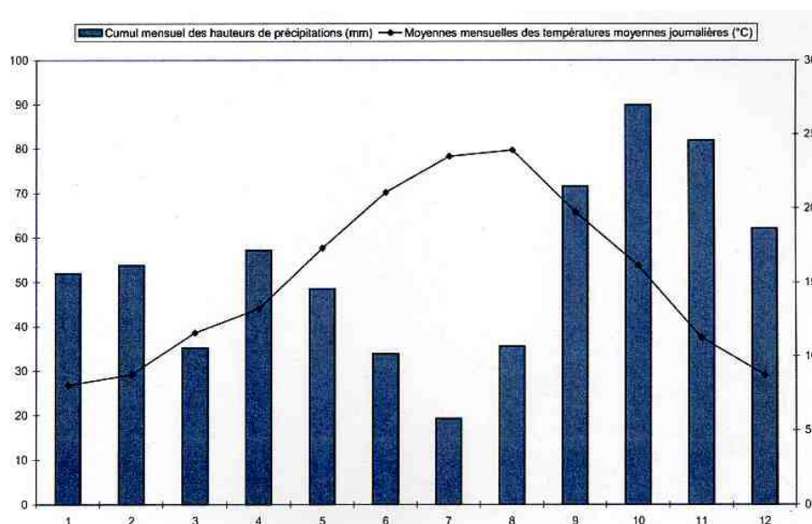
Figure 4 : Diagramme ombrothermique moyen sur la période 1989 - 2005.
