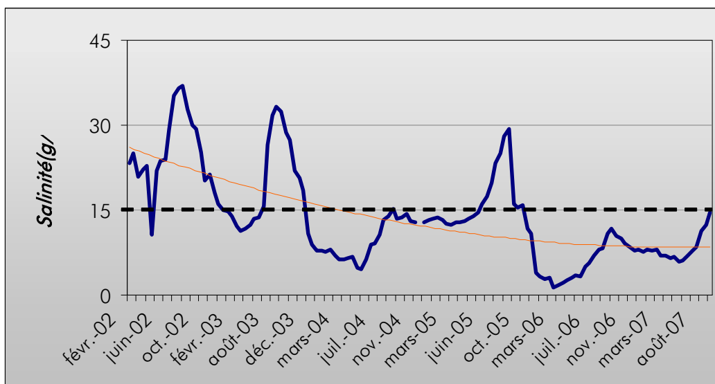
Fig. 1 : Evolution de la salinité de l'étang de Vendres 2002-2007
